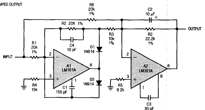
Precision Rectifier
