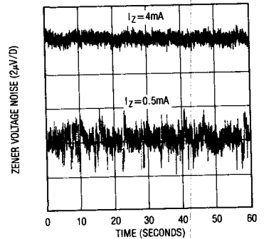
Zener Noise
