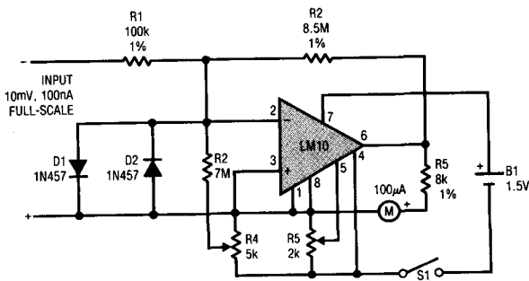
Meter Amplifier
