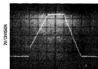
A_V = +1 , 20\mu sec/DIV
